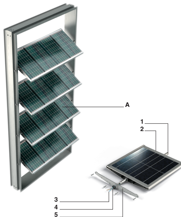
A - Lamella con pannello fotovoltaico
