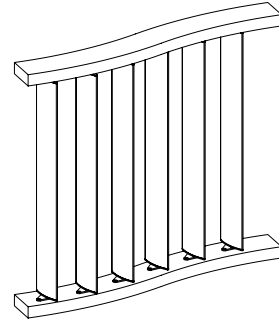
D12 - Frangisole verticale per sottostruttura. Angoli prestabiliti.
